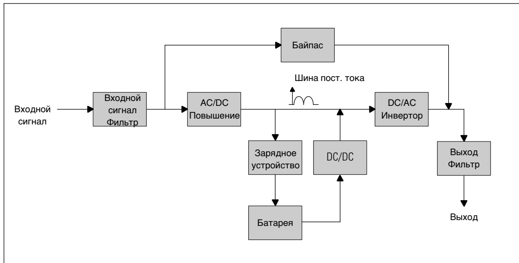
Рисунок 27. 5600W Блок-схема линейно-интерактивного ИБП
