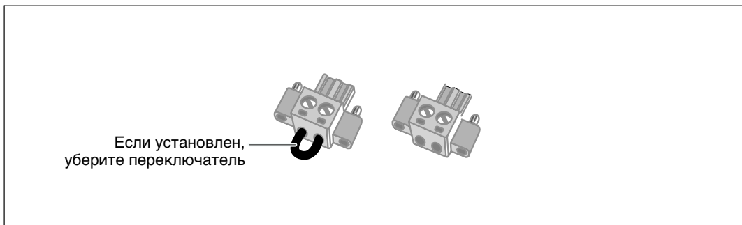
Рисунок 16.Соединитель REPO
