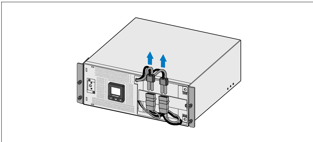
Рисунок 25. Отсоединение разъемов внутренних батарей
