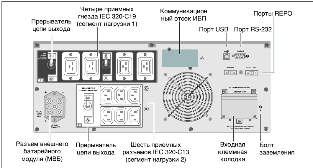
Рисунок 5. Задняя панель 5600W, 230 В
