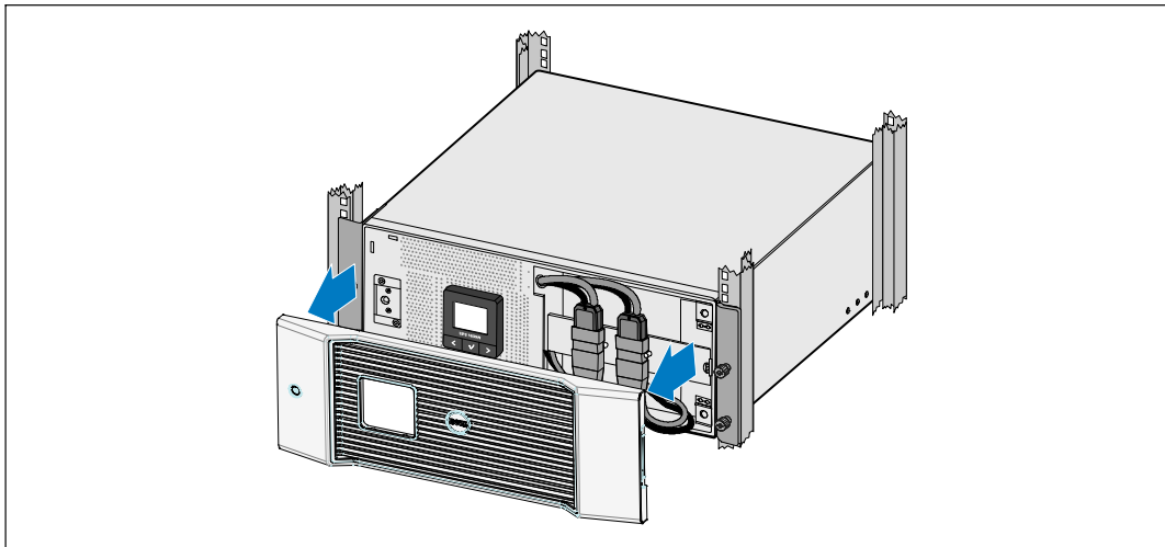
Рисунок 24. Снятие передней крышки ИБП
