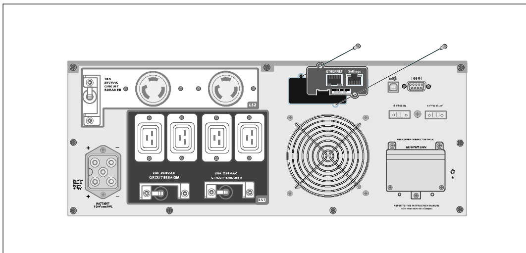
Рисунок 23. Карта сетевого управления Dell
