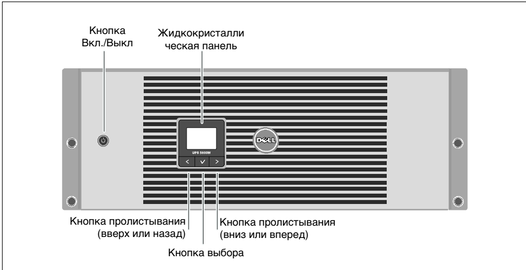
Рисунок 6. Передняя панель ИБП Линейно-интерактивный, монтируемый в стойку Dell
