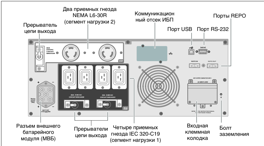
Рисунок 4. Задняя панель 5600W, 208 В
