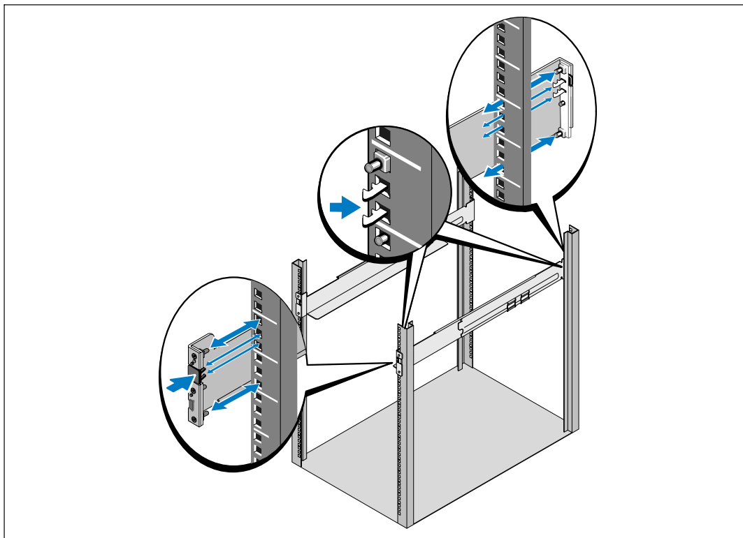
Рисунок 9. Установка реек
